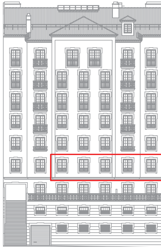
ALÇADO POSTERIOR
